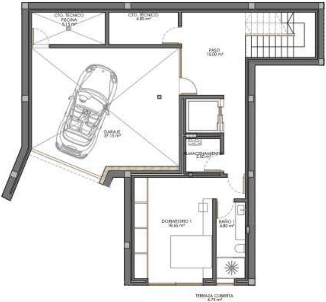
Planta Sótano
