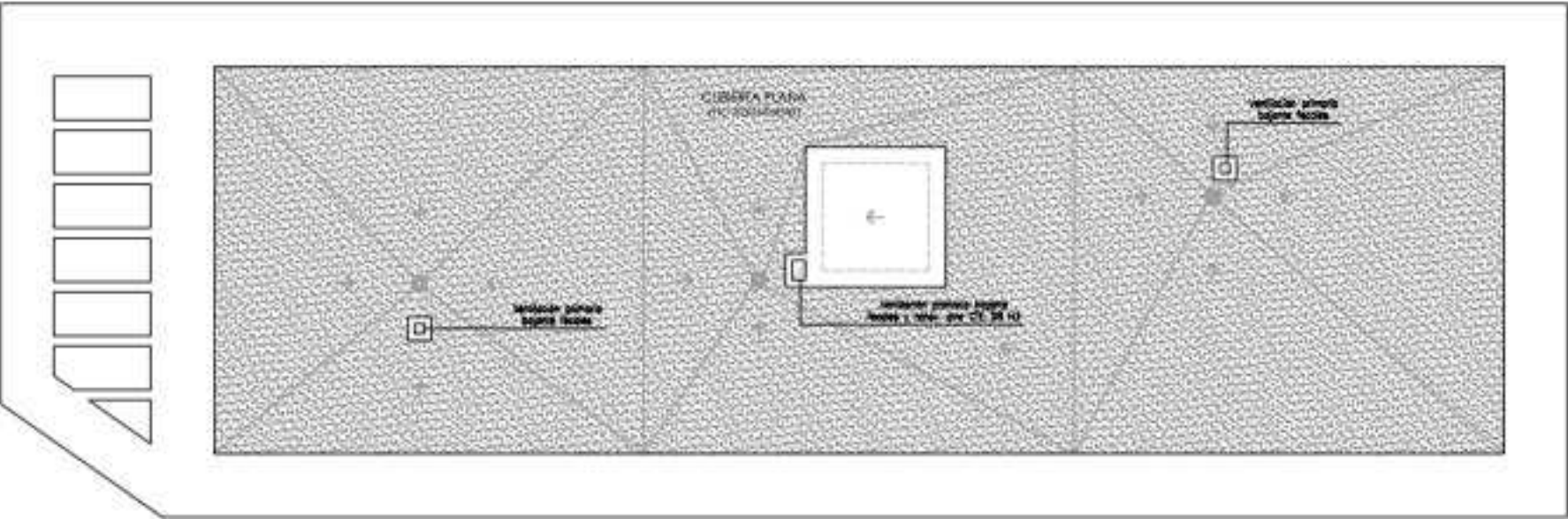
Planta Cubierta
